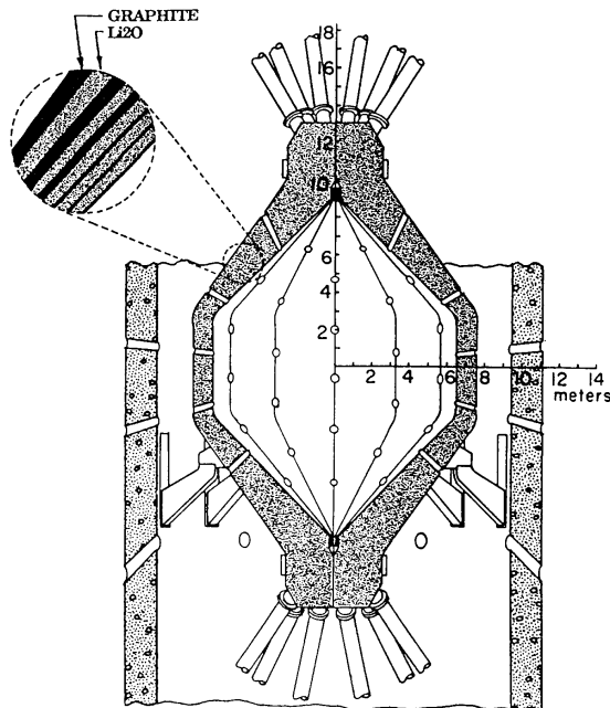
SOMBRERO (1992)
